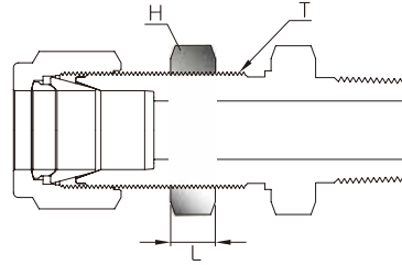
Metric tube OD
